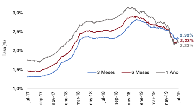
Tasas LIBOR
