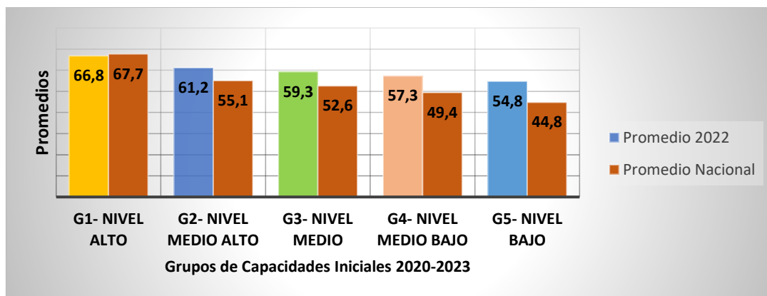
Gráfica 4 Promedio de la puntuación de gestión por capacidades iniciales 2022
