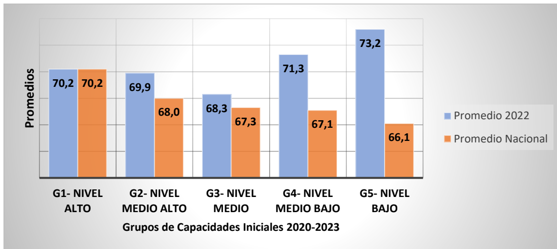
Gráfica 10 Promedio de la puntuación de resultados por capacidades iniciales 2022
