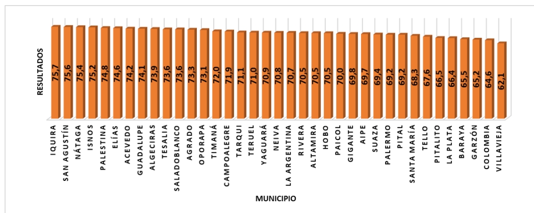
Gráfica 9 Posición de los municipios en el componente de resultados
