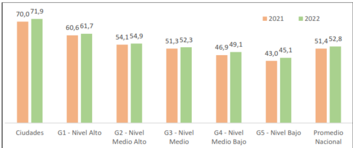
Gráfica 15 Promedio de la puntuación de MDM nacional por capacidades iniciales 2021-2022
