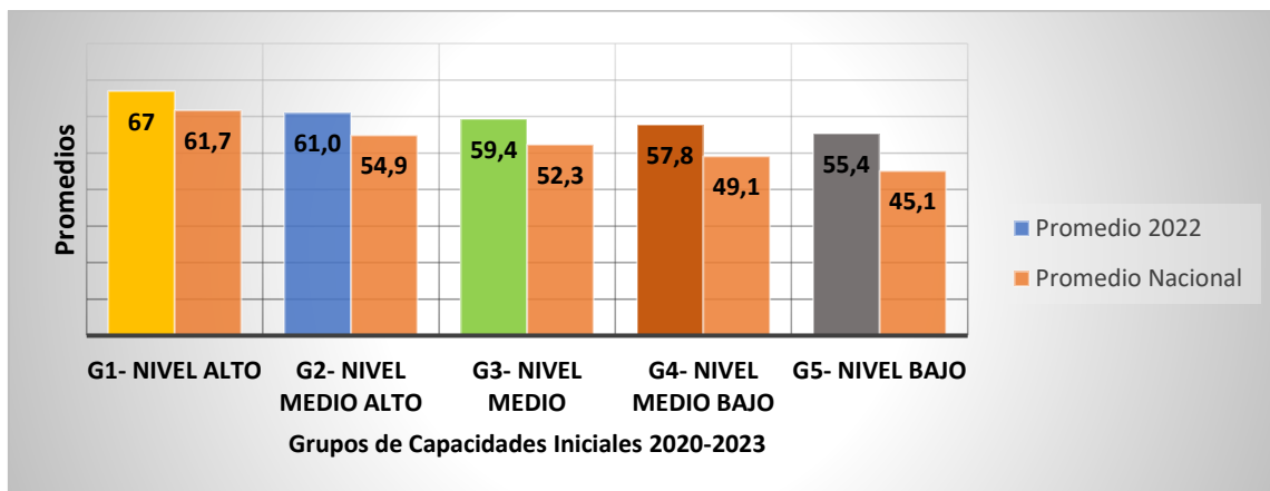
Gráfica 13 Promedio de la puntuación de MDM por capacidades iniciales 2022.
