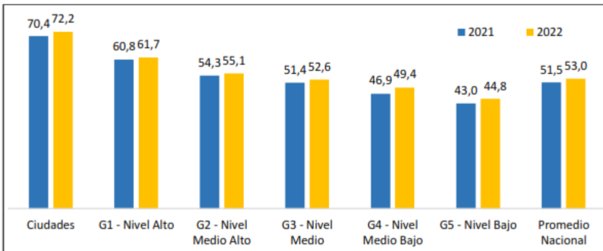
Gráfica 6 Promedio nacional de la puntuación de gestión por capacidades iniciales 2021-2022
