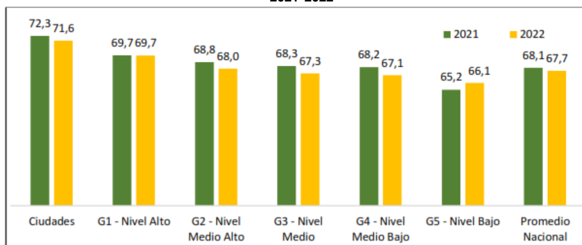
Gráfica 12 Promedio de la puntuación de resultados nacionales por capacidades iniciales 2021-2022
