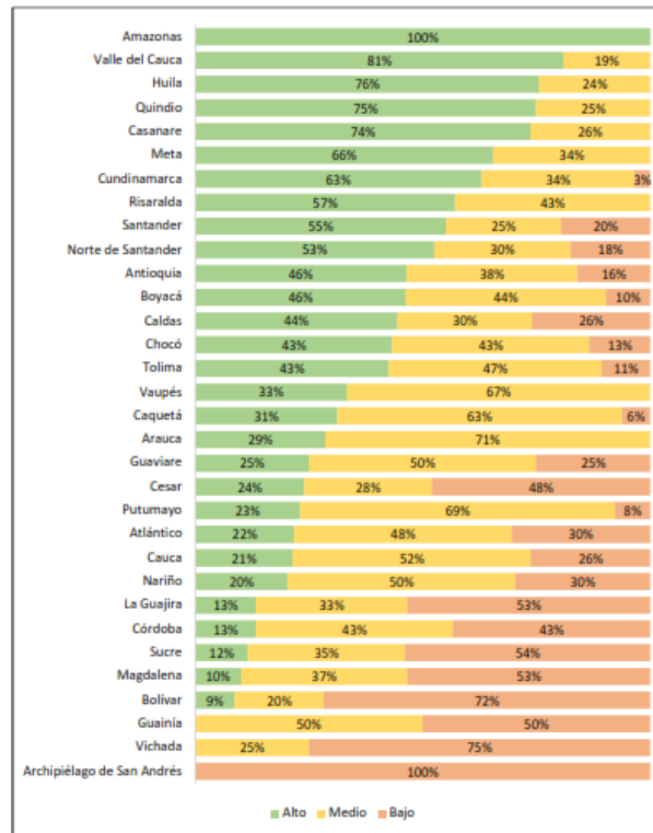
Gráfica 17 Porcentaje de municipios en calificación Alta, Media y Baja MDM por departamento.
