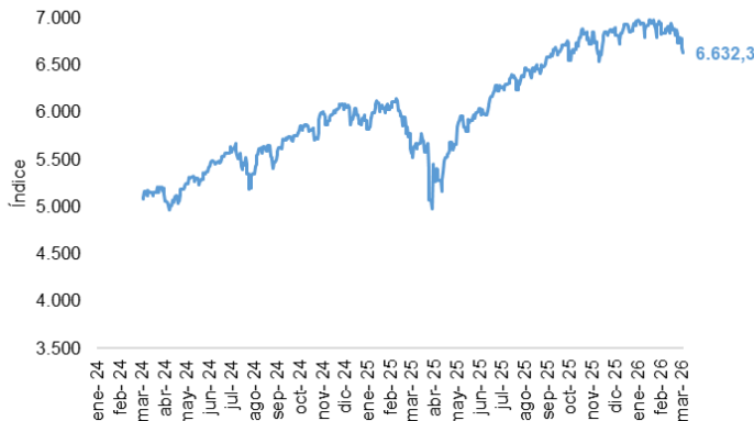
Índice S&P 500
