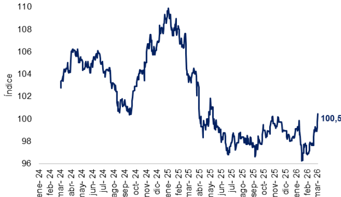
Índice DXY
