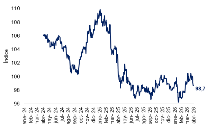
Índice DXY
