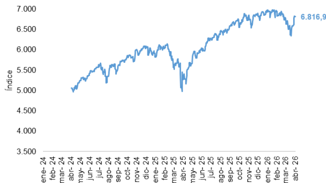
Índice S&P 500
